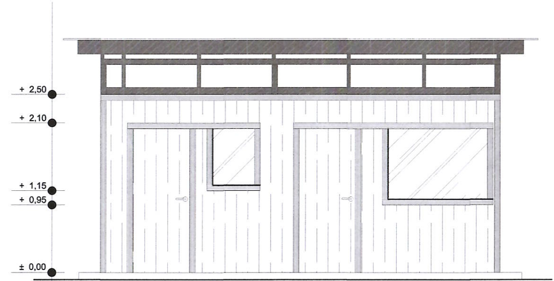
TAMPAK DEPAN GUDANG SKALA 1 : 50
