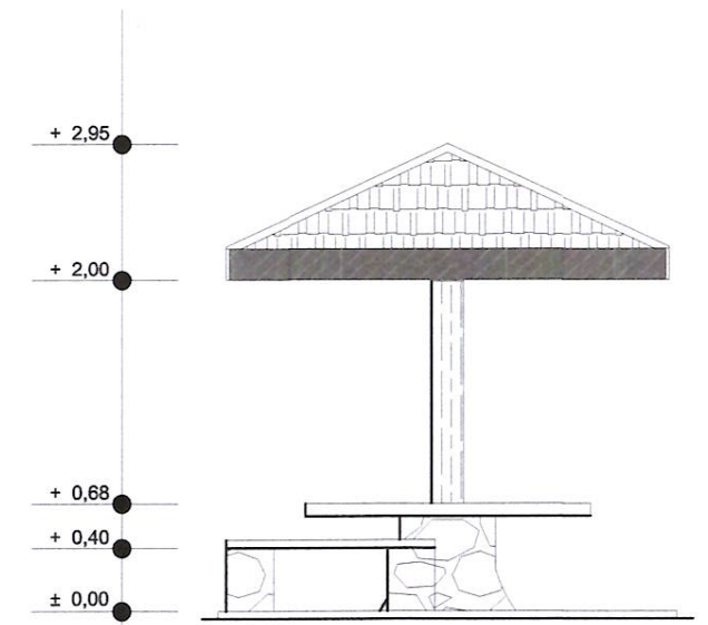
TAMPAK GAZEBO SKALA 1 : 50
