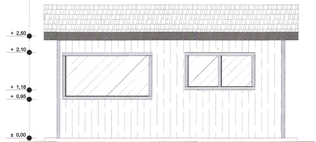
TAMPAK BELAKANG GUDANG SKALA 1 : 50
