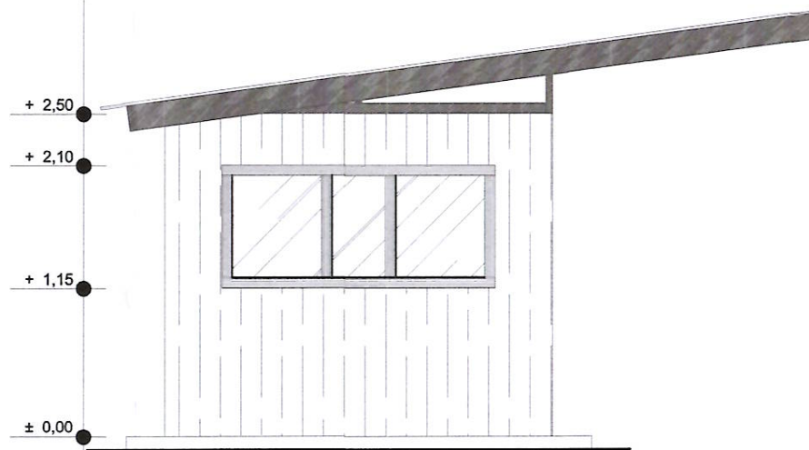
TAMPAK SAMPING KIRI GUDANG SKALA 1 : 50
