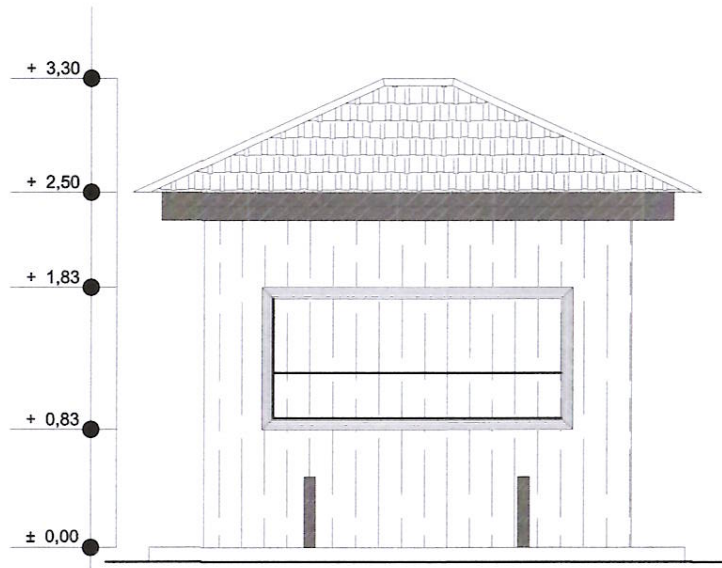
TAMPAK DEPAN BOOTH SKALA 1 : 50
