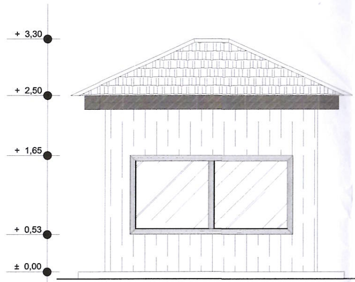
TAMPAK BELAKANG BOOTH SKALA 1 : 50
