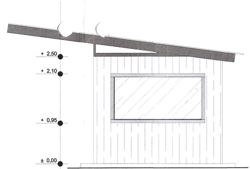
TAMPAK SAMPING KANAN GUDANG SKALA 1 : 50
